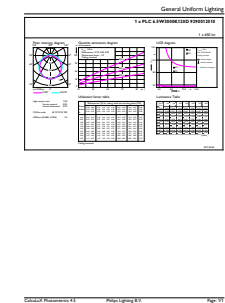
LEDtube PLC 100mm 7W G24Q-2 830 650lm
