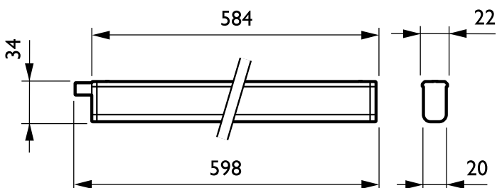
Pentura Mini BN130C-BN133C
